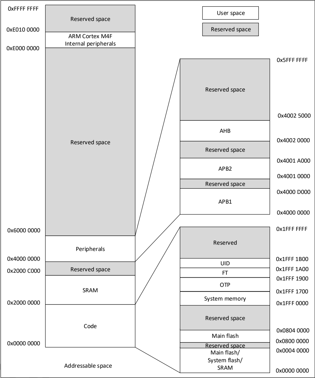
图 4-1 存储器映射
