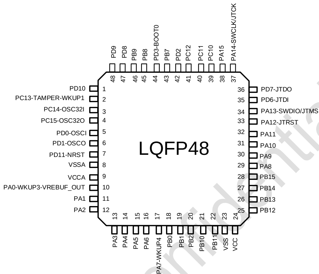
图 3-2 LQFP48 PY32F42xC2xT7 Pinout2 (Top view)
