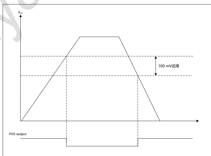
图 2-4 PVD 阈值
