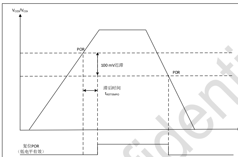
图 2-3 POR/PDR 阈值
