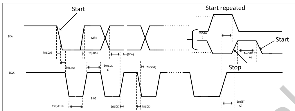
图 5-3 I²C 总线时序图
