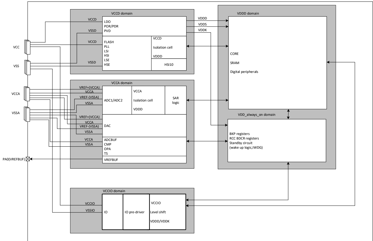
图 2-2 电源框图
